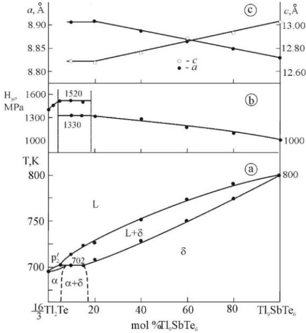
Şəkil 1. Tl 2 Te-Tl 9 SbTe 6 sisteminin faza diaqramı (a), mikrobərkliyin (b) və qəfəs parametrlərinin (c) tərkibdən asılılıqları
