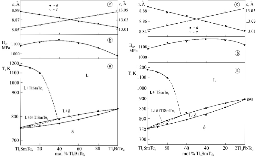
Şəkil 7. Tl_9SmTe_6 - Tl_9BiTe_6 və Tl_9SmTe_6 - Tl_9PbTe_6 sistemlərinin faza diaqramı (a), mikrobərqliyin (b) və kristal qəfəs parametrlərinin (c) tərkibdən asılılıqları.
