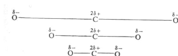
Рис. Симметричное валентное колебание \text{CO}_2
