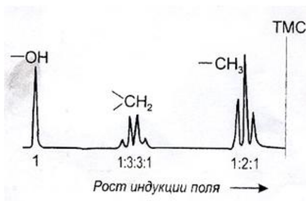
Рис. 1. Спектр ЯМР высокого разрешения подкисленного этанола.
