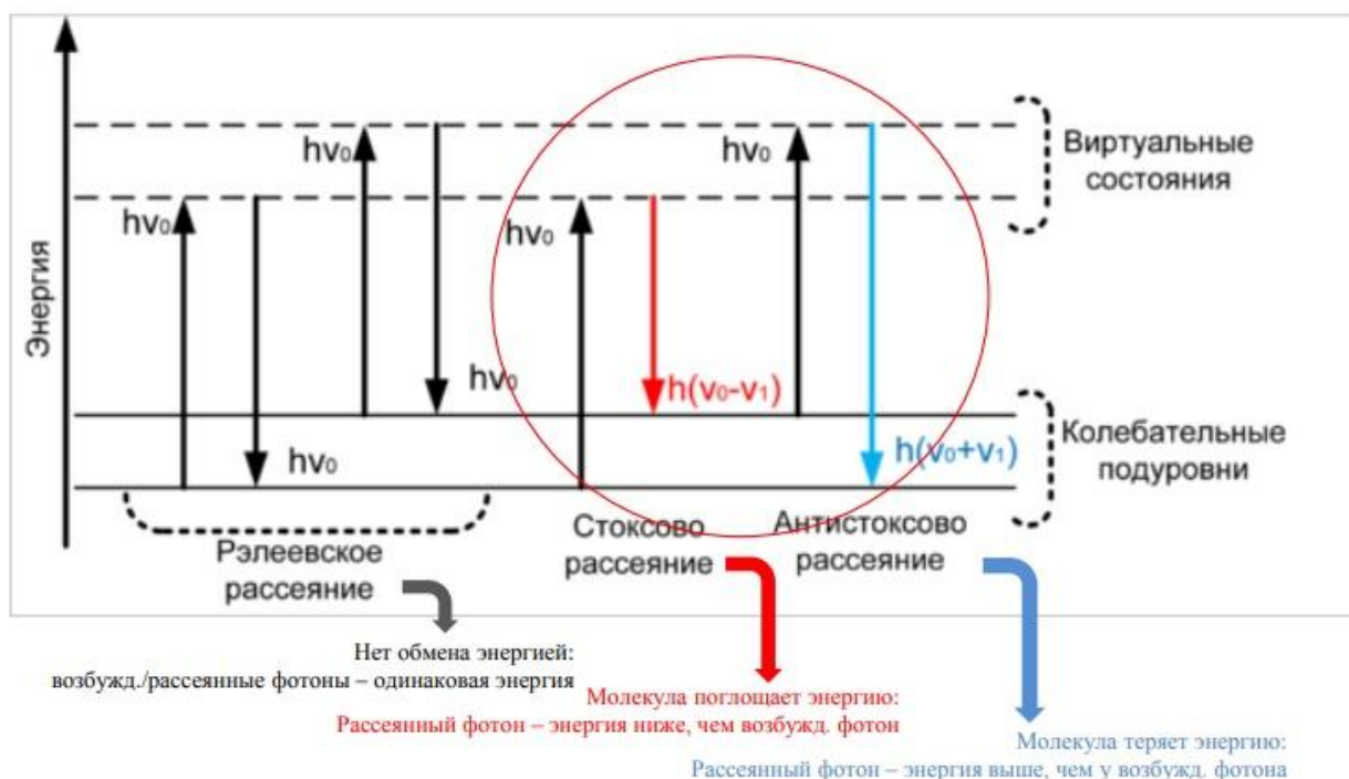
Рисунок. Эластичное (релеевское) и комбинационное (рамановское) рассеяние света
