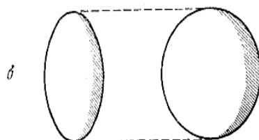
Вид молекулы водорода и ее эллипсоида поляризуемости в двух взаимно перпендикулярных направлениях.
