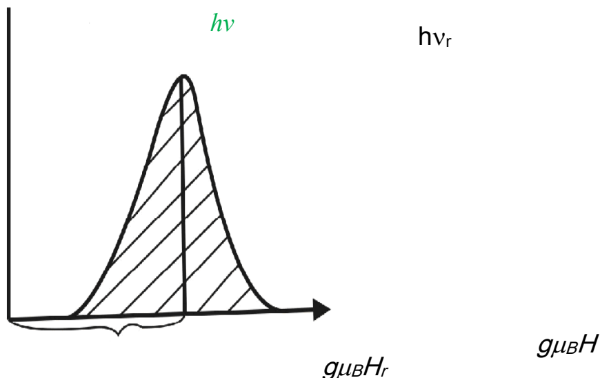
Рисунок. Зависимость энергии резонансного поглощения от энергии постоянного магнитного поля.
