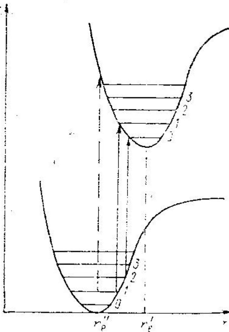
Электронно-колебательные переходы при учете принципа Франка-Кондона для внутримолекулярных процессов.
